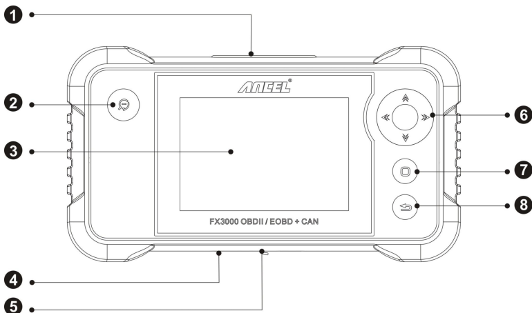
Figure 3-1 Vue avant du FX3000
